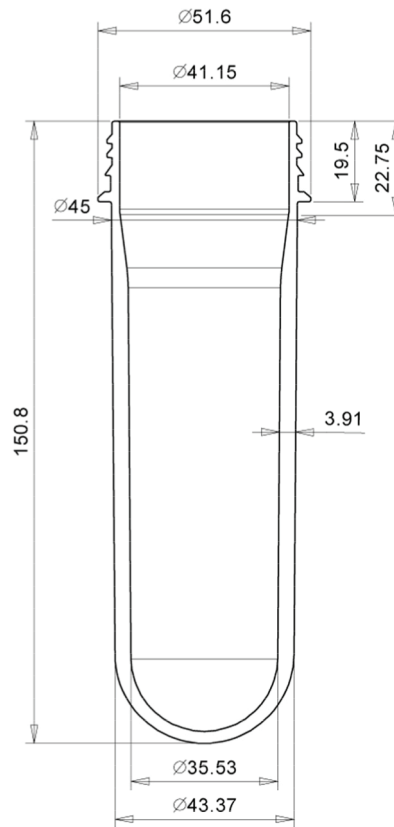
A-A View/Görünüm
